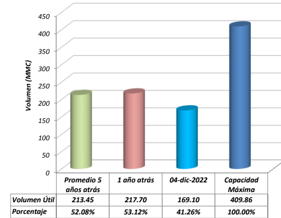
COMPARACION DE VOLÚMENES Sistema Hidráulico Chili
