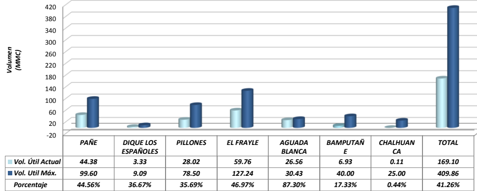
VOLÚMENES DE REPRESAS Sistema Hidráulico Chili
