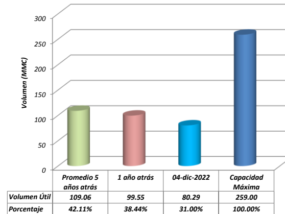
COMPARACIÓN DE VOLÚMENES Sistema Hidráulico Colca
