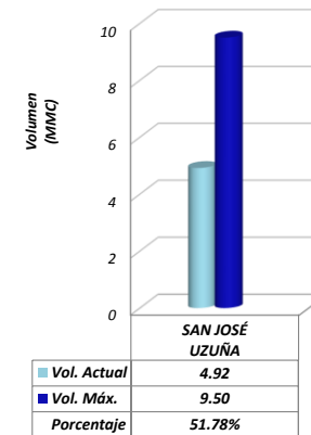
VOLUMEN DE REPRESA CUENCA ORIENTAL San Jose de Uzuña
